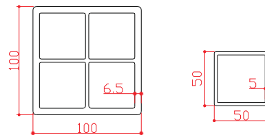
3. 方管 Square pipe
